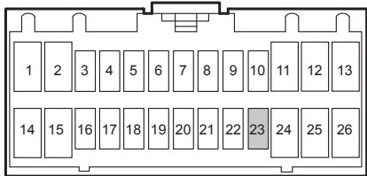
IP93 PEPS ECU 1 线束连接器
