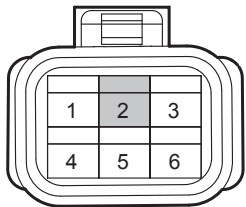
EN28b 变速器档位开关线束连接器
