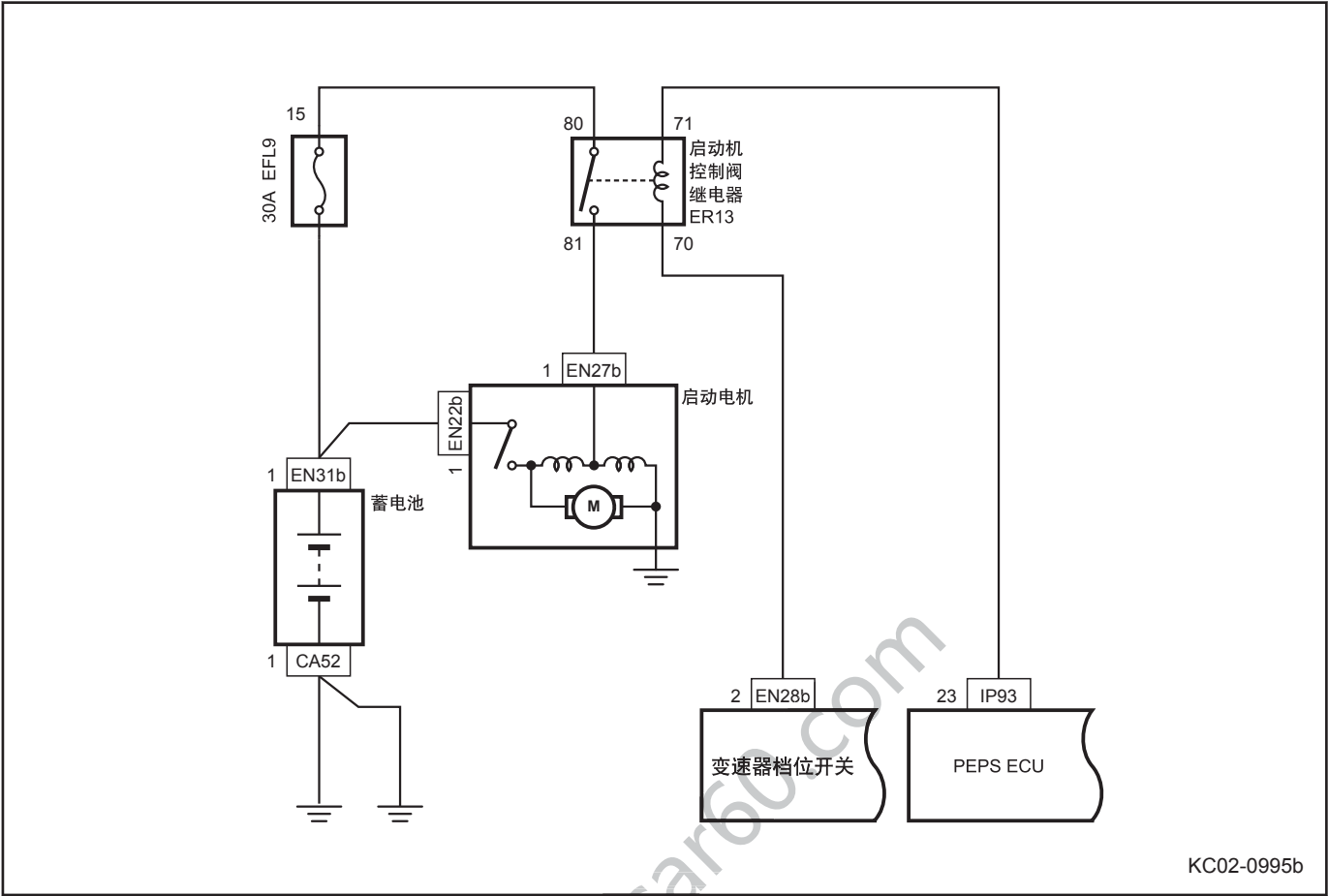
启动系统原理图
