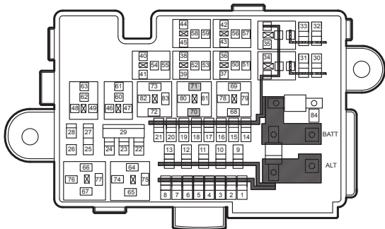
CA01 发动机舱保险丝继电器盒
